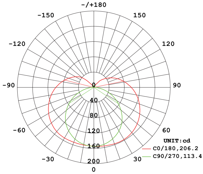
配光曲线
